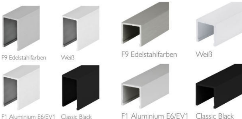
Profil für Decke und Wand 44 x 25 25 x 25
