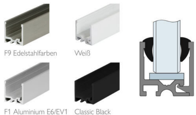
Profil für Boden und Wand 25 x 25
